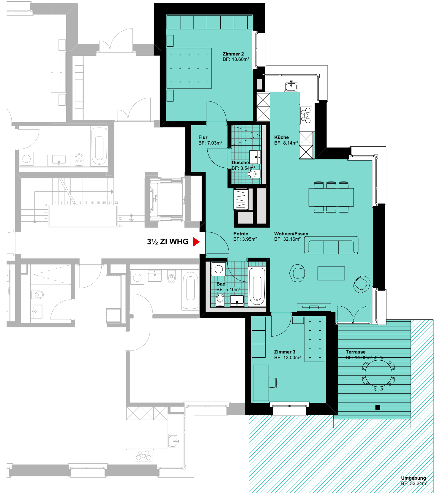
Grundriss Wohnung
