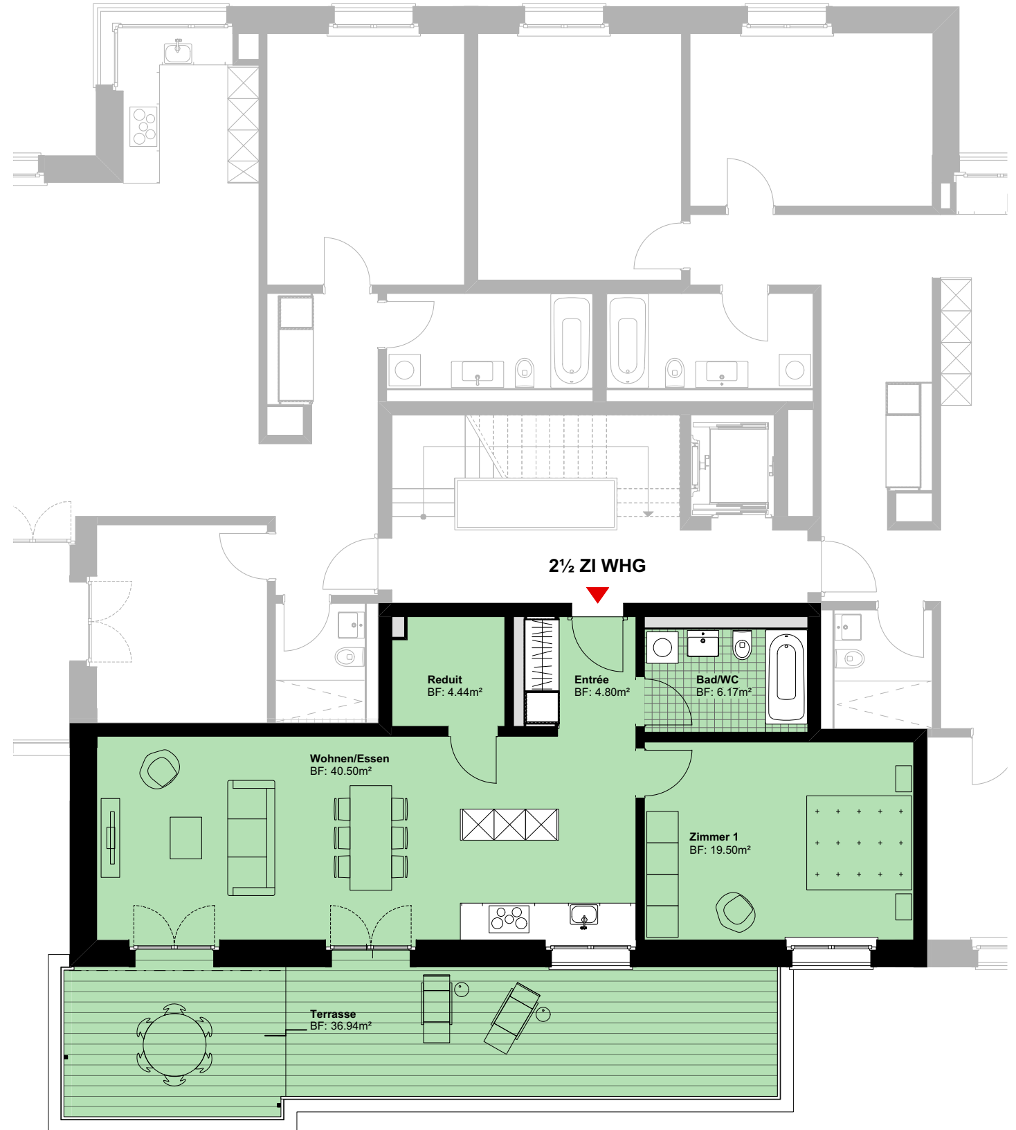
Grundriss Wohnung
